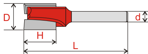
Схема основных габаритов фрез
